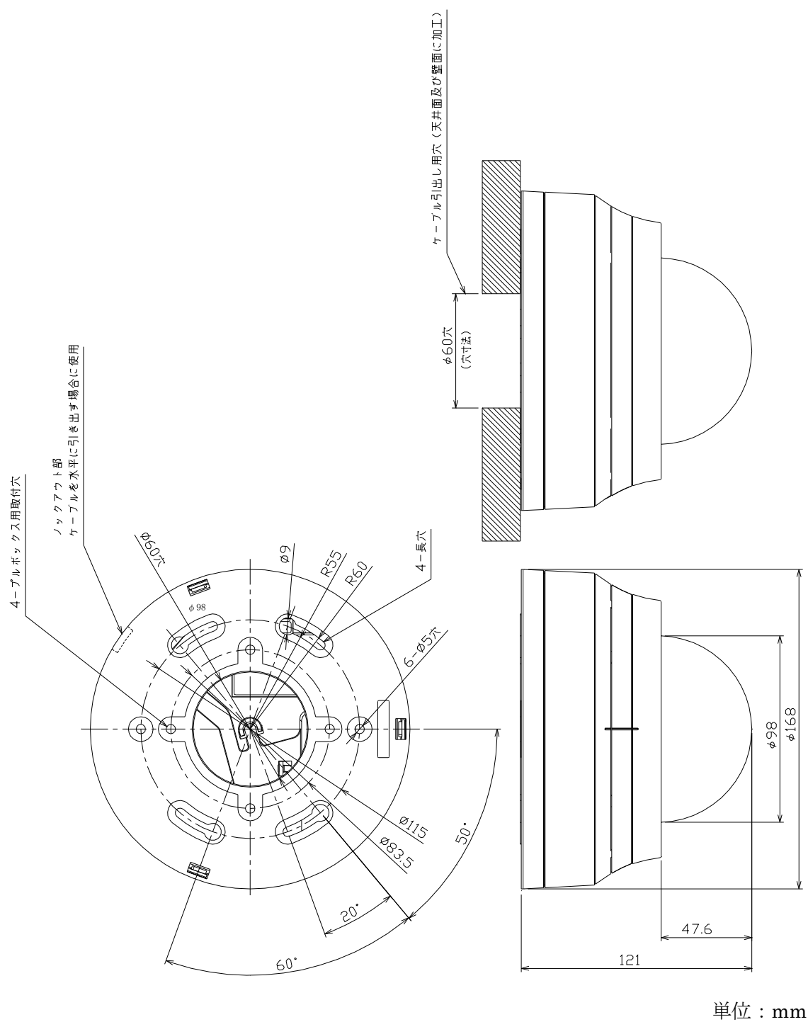
図 15-1 外形図
